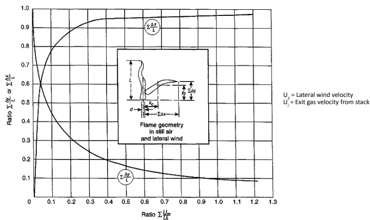
FIGURA 6 - Distorção chama devido à velocidade lateral do vento e do jato de gás. Fonte API RP 521
