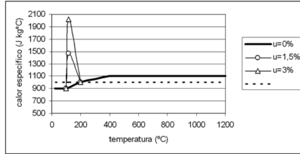
FIGURA 9 - Calor específico do concreto
