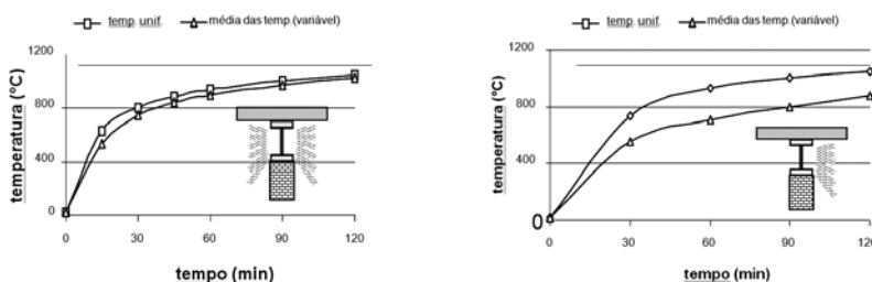
FIGURA 40 - Temperatura no aço determinada por método analítico e numérico (Supertempcalc), para: a) fogo em duas faces b) fogo em uma face
